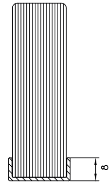
Optional end cap profile Profilé optionnel raccord
