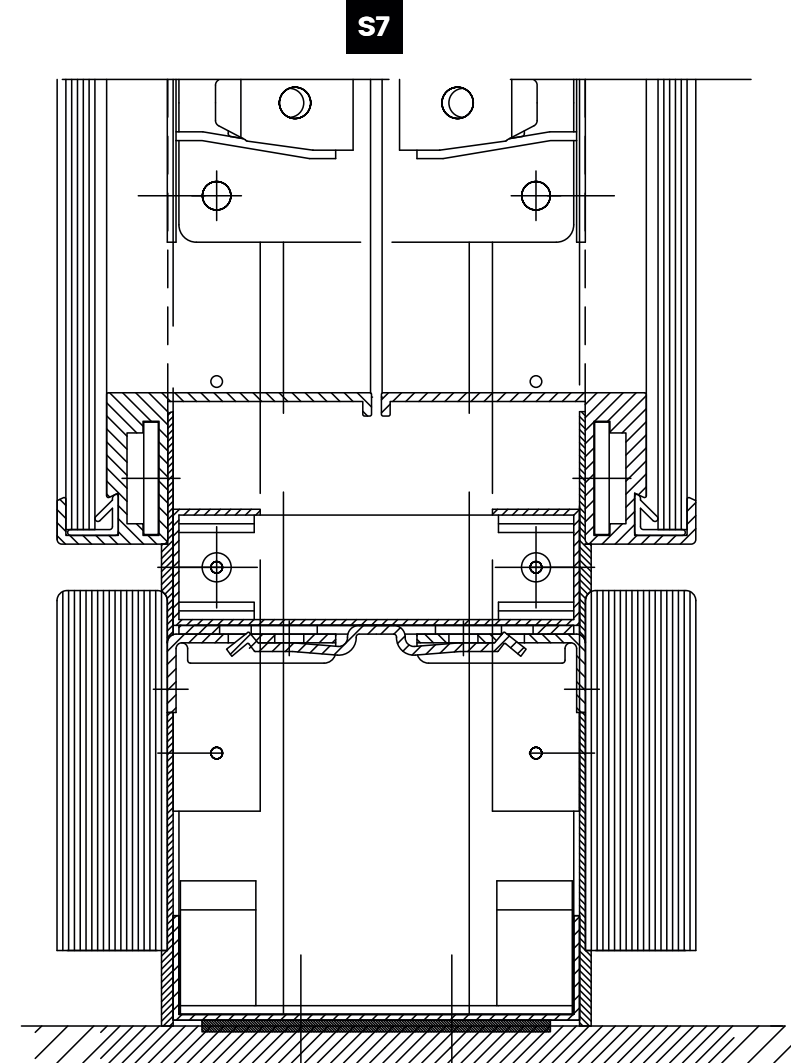
Optional end cap profile Profilé optionnel raccord
