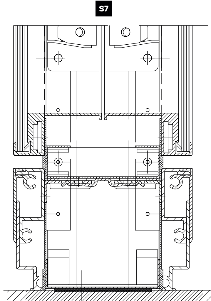
Zócalo de aluminio regulable
