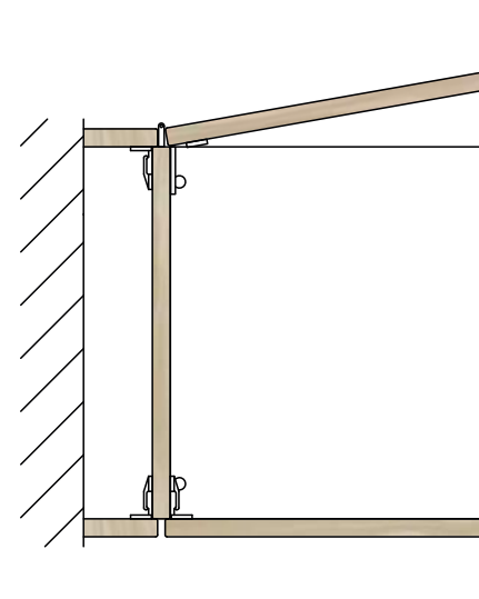
Arranque de pared con remates Wall starter of wall with end caps Départ de mur avec raccords
